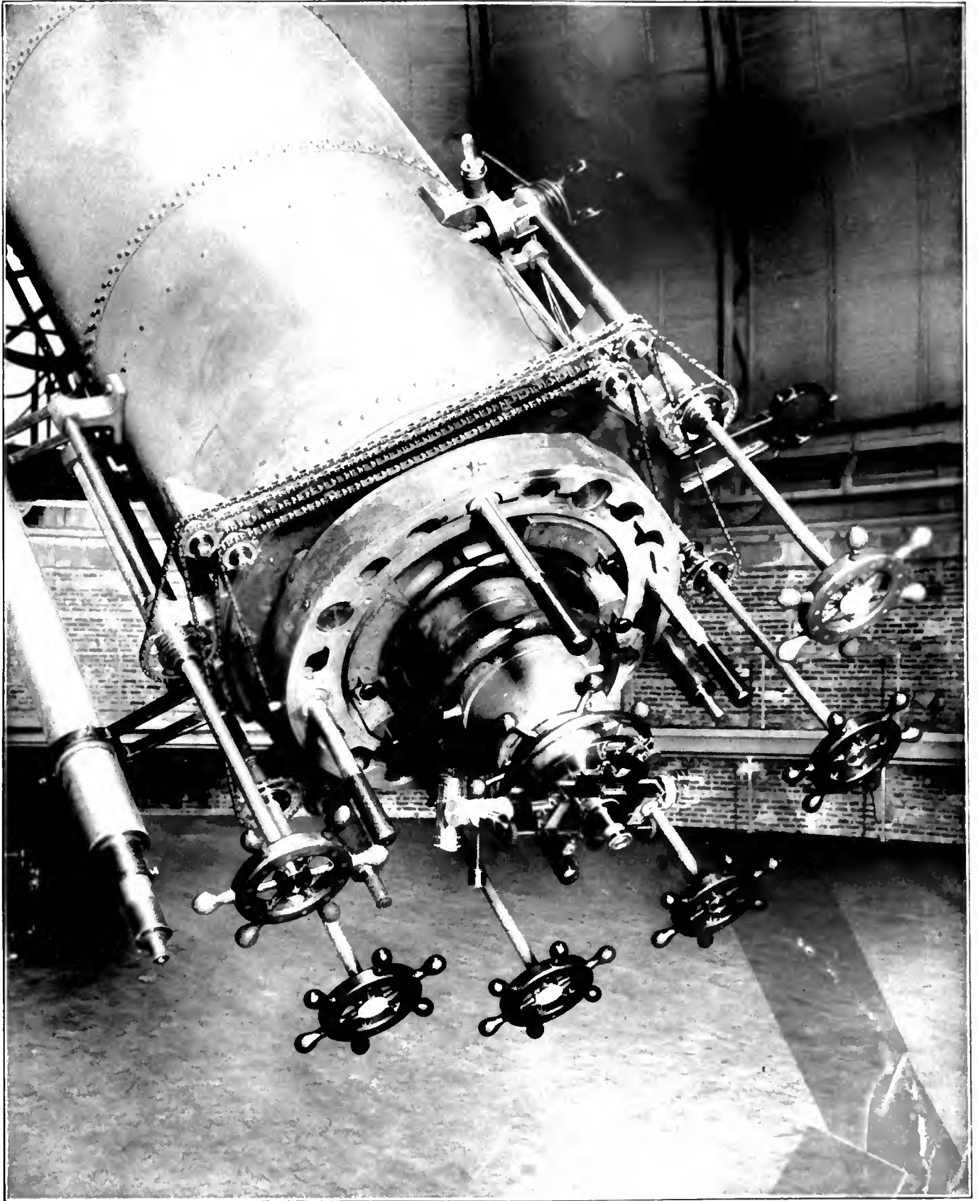
FIG. 25.—EYE END OF 40" YERKES TELESCOPE.
