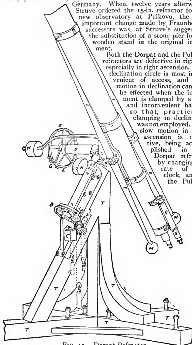
FIG. 13.—Dorpat Refractor.
