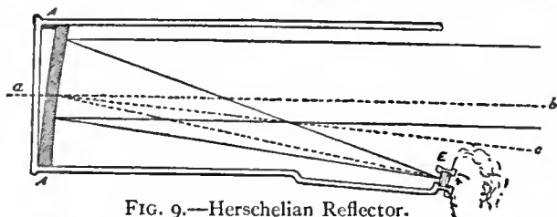
FIG. 9.—Herschelian Reflector.
